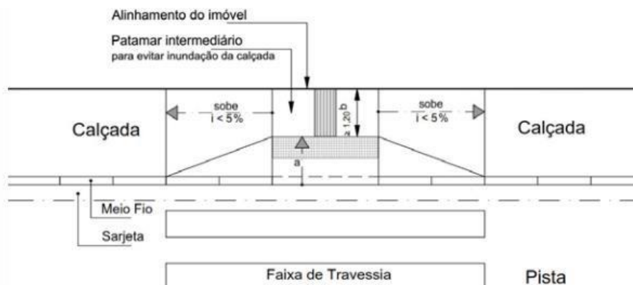
Imagem 01 – Modelo de rampa para Calçadas com dimensões menores de 2,60 metros. Fonte: NBR 9050/2020
